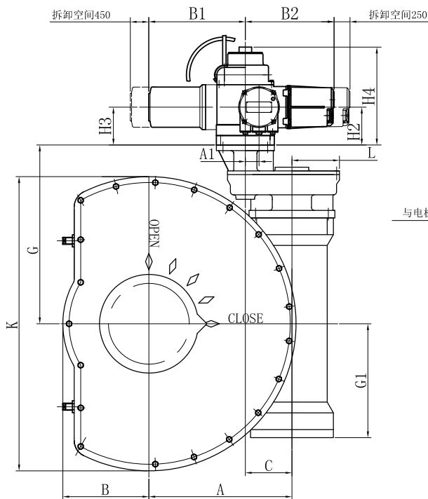
IMC100~300带HAJBC系列外形及连接尺寸
